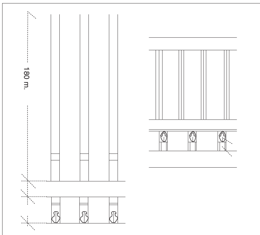
Detalles del Coro de Masegoso (planta y alzado) 38
