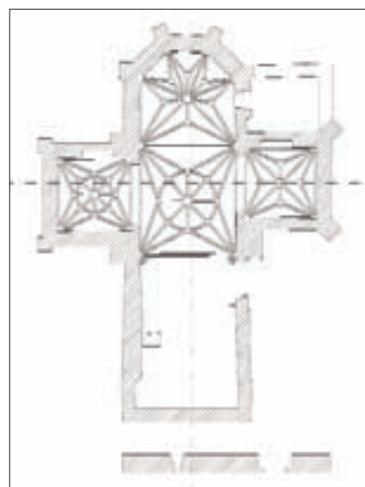
Planta de techumbres, con la que podría ser la cubierta del presbiterio hundida en los años 60 del pasado siglo.
