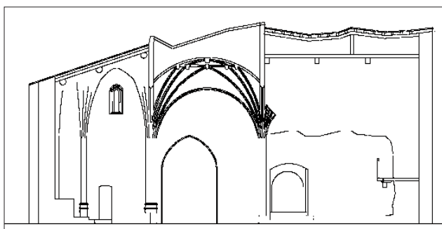
Sección longitudinal hacia el sur con la entrada y la conexión con la capilla más primitiva con arco ojival rebajado sin decoración alguna.
