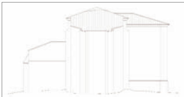
Planos del alzado Este donde se aprecia la diferente altura de las dos capillas laterales.
