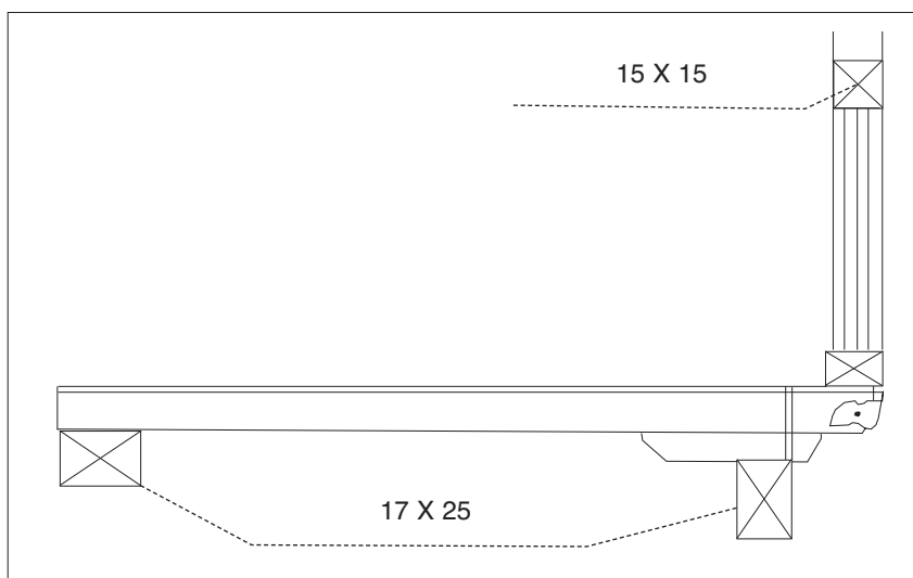
Sección del Coro de Masegoso 37
