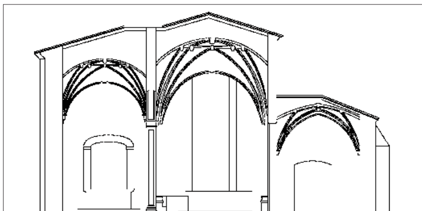
Sección transversal por las capillas hacia el presbiterio donde se aprecia la diferente altura y decoración de cada capilla.
